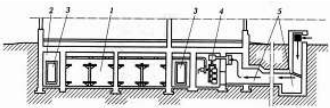
Рис. 1.2. Противорадиационное укрытие: 1 — отсеки для укрываемых людей; 2 — тамбур; 3 — защитно-герметические двери; 4 — фильтровентиляционная установка; 5 — аirtightный выход, используемый для забора воздуха
