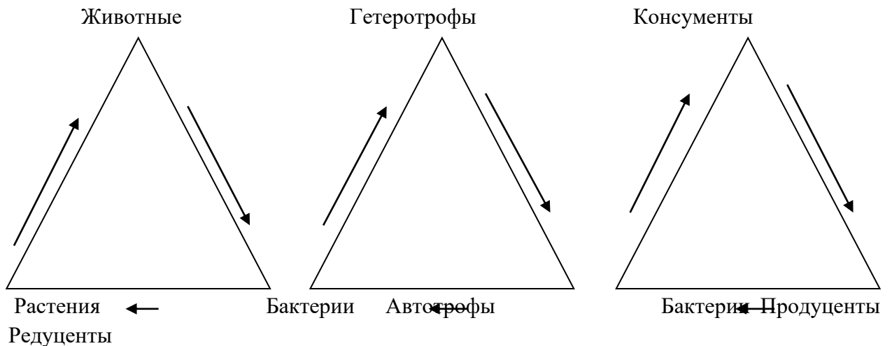
Круговорот веществ и энергии в пищевых цепях.
