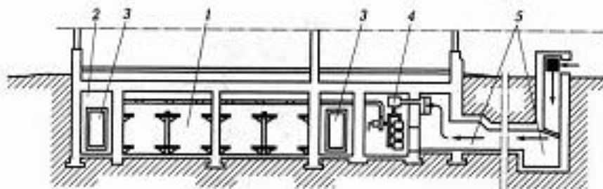
Рис. 1.2. Противорадиационное укрытие:
