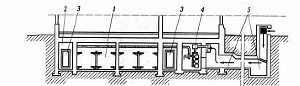
Рис. 1.2. Противорадиационное укрытие: 1 — отсеки для укрываемых людей; 2 — тамбур; 3 — защита-герметические двери; 4 — фильтровентиляционная установка; 5 — аварийный выход, используемый для забора воздуха
