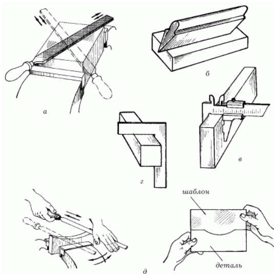
Рис. 2 – Опиливание поверхностей и контроль за качеством работ: а – перекрестное опиление; б – контроль отклонений от плоскости и прямолинейности; в – контроль отклонений от параллельности; г – контроль отклонений от перпендикулярности; д – контроль криволинейных поверхностей по шаблону.
