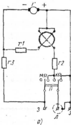
Рис. 1. Измерение сопротивления изоляции: а — схема соединений мегомметра М-1101. б — схема присоединения испытуемого провода к мегомметру.
