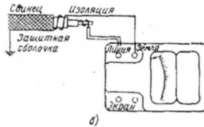
Рис. 1. Измерение сопротивления изоляции: а — схема соединений мегомметра М-1101. б — схема присоединения испытуемого провода к мегомметру.
