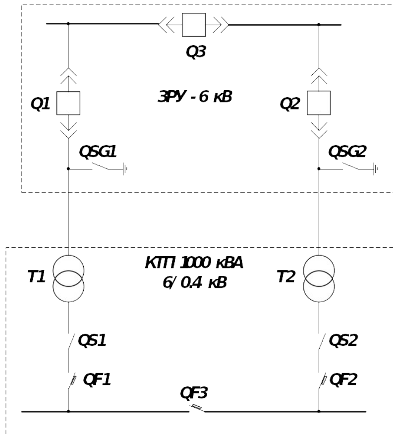
Рисунок 1 – Принципиальная электрическая схема КТП 1000 кВА
