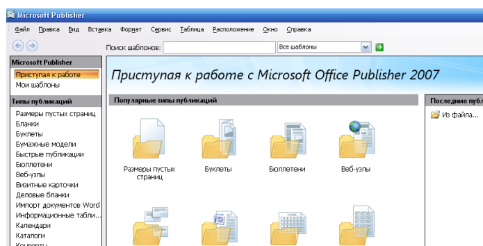
Рис. 1. Интерфейс программы.
